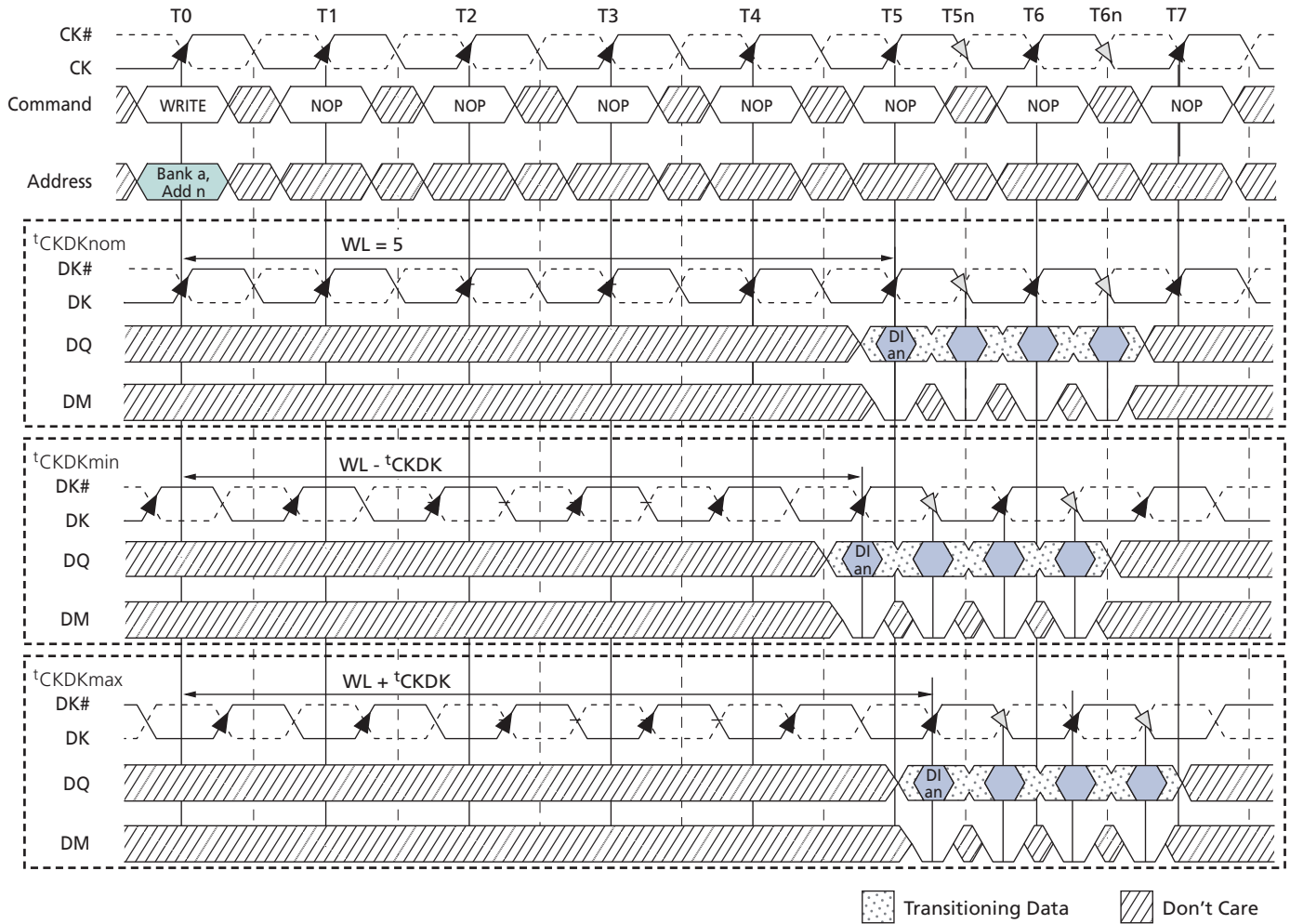
Figure43: WRITE Burst
